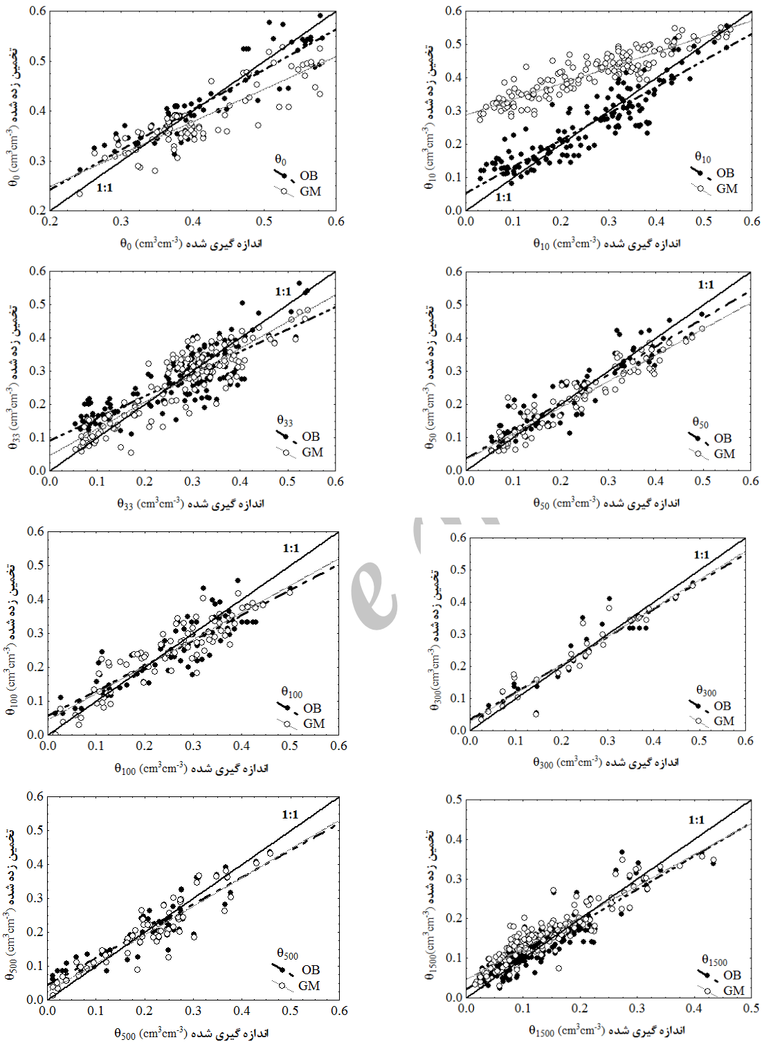
شکل ۳ - مقایسه برآورد رطوبت در مکش‌های مختلف توسط دو گروه توابع انتقالی با مقادیر اندازه‌گیری شده برای داده‌های اولیه. خط ممتد خط ۱:۱ است. OB توابع پیشنهادی و GM توابع فنی‌رسان - میلان (۲۰۱۰) است.
