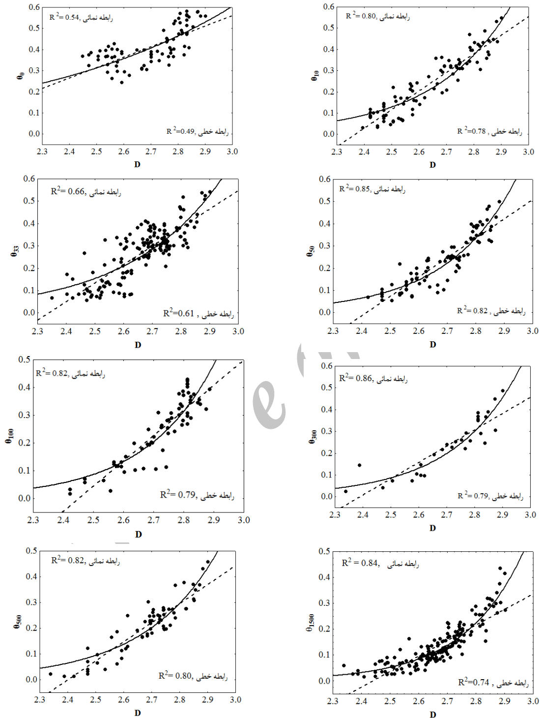
شکل ۲- نمودارهای پراکنش رطوبت در نقاط مختلف منحنی رطوبتی در مقابل بعد فرکتال بافت خاک به همراه یک رابطه‌ی خطی ( \theta = b_0 + b_1 D ) و یک رابطه‌ی نمایی ( \theta = \exp(b_0 + b_1 D) ) که به هر نمودار تحمیل شده است.
