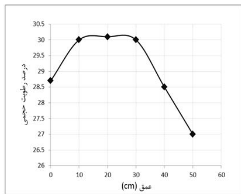
شکل ۱۰- درصد رطوبت حجمی در جهت عمودی در راستای قرارگیری قطره‌چکان ۴۸ ساعت بعد از آبیاری، (a) شبیه‌سازی شده، (b) اندازه‌گیری شده
