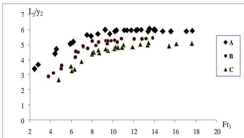
شکل ۹- تغییرات طول بی‌بعد پرش هیدرولیکی در برابر عدد فرود اولیه
