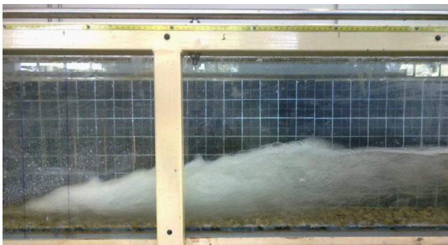
شکل ۸- نمایی از پرش هیدرولیکی در بستر زبر ۳/۵ میلی‌متر
