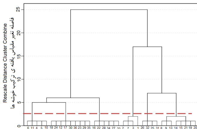
شکل 6- دندوگرام حاصل از خوشه‌بندی لایه ی کوهونن با استفاده از الگوریتم وارد و فاصله اقلیدسی
