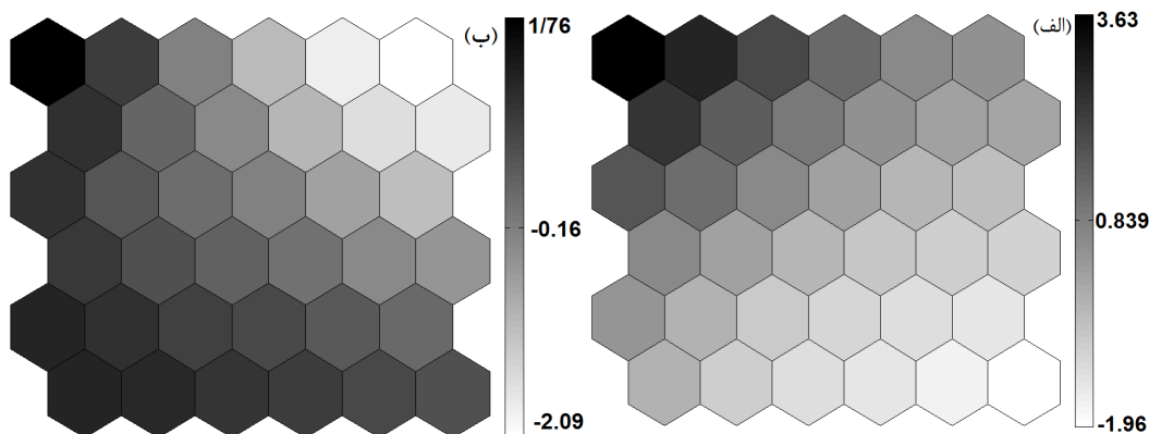
شکل 5- توزیع مولفه اول (الف) و مولفه دوم (ب) در نقشه آموزش یافته SOM (رنگ تیره نشان دهندهی مقایر زیاد هر مولفه و رنگ سفید کمترین مقدار را نشان می‌دهد).
