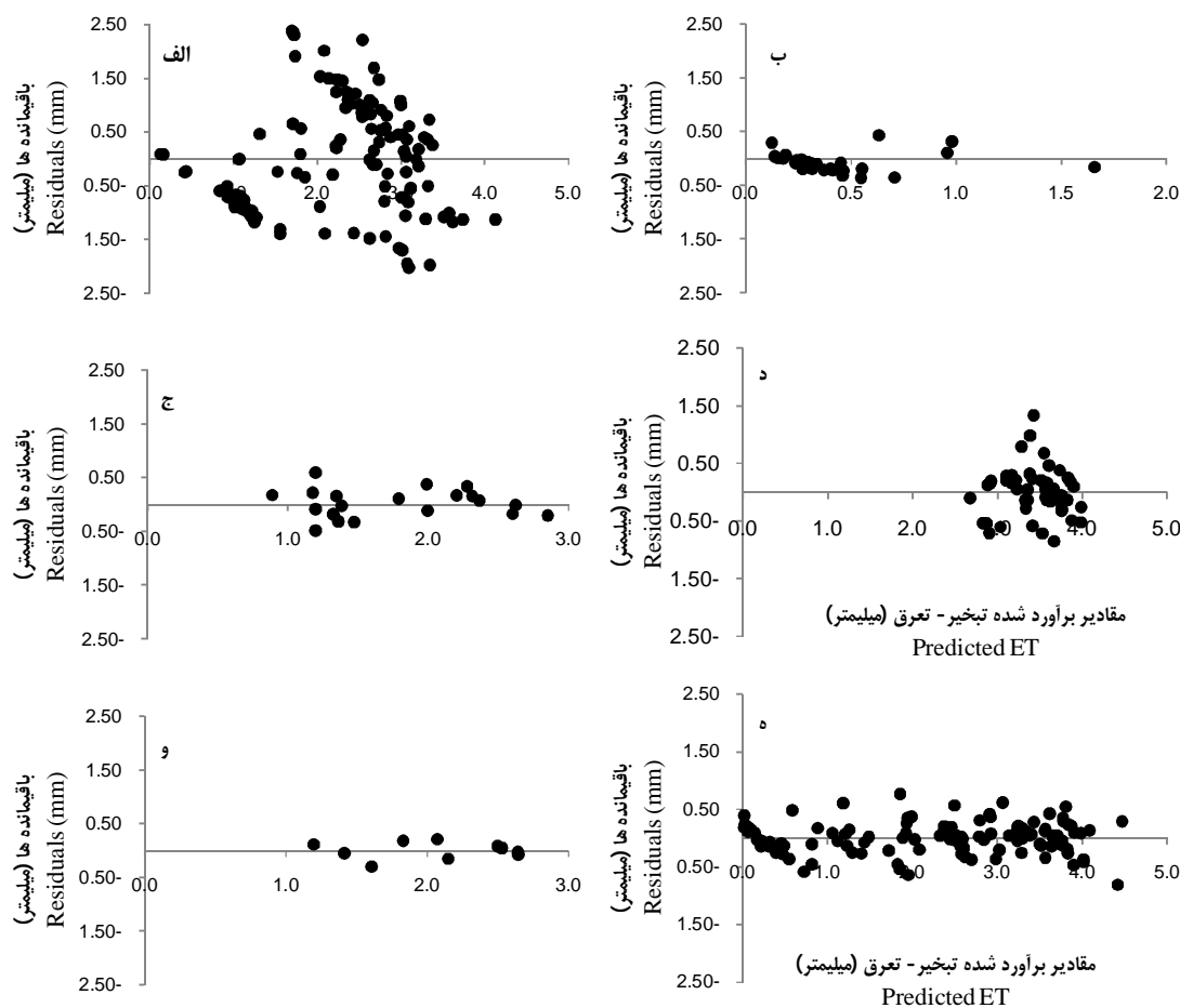
شکل 5- مقادیر باقیمانده و برآورد شده تبخیر - تعرق در رگرسیون؛ (الف) تمام دوره رشد، (ب) مرحله ابتدایی رشد، (ج) دوره دوم، (د) دوره سوم، و (ه) دوره انتهایی رشد و (ه) شبکه عصبی
