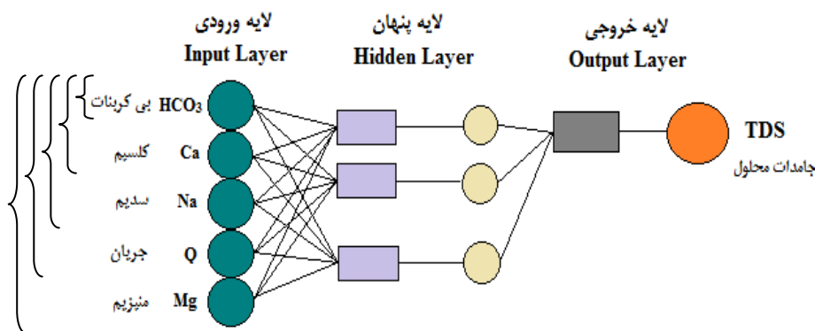
شکل ۲- نمودار شماییک یک شبکه عصبی چند لایه با ورودی‌های مدل Figure 2- ANN structure with inputs of model
