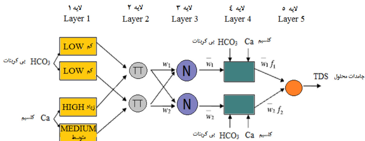
شکل ۳- نمای شماییک مدل سامانه استنتاجی عصبی-فازی تطبیقی Figure 3- Adaptive neuro-fuzzy inference systems structure
