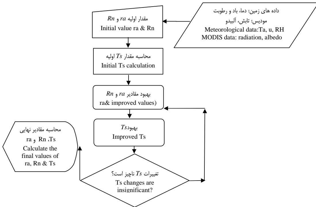
شکل ۴- فلوجارت فرآیند تکرار برای محاسبه دمای سطح زمین Figure 4- Iterative flowchart for surface temperature(Ts) calculation
