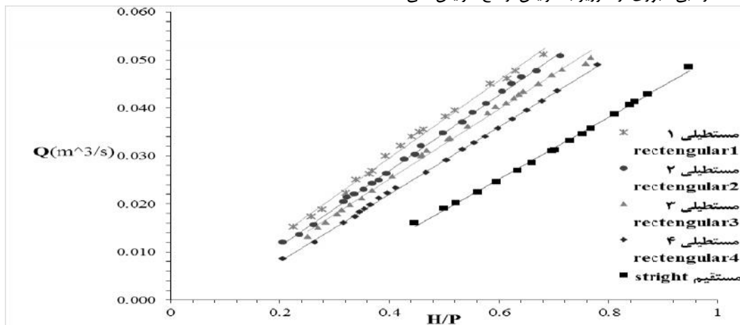
شکل ۳- نمودار تغییرات دبی در برابر نسبت H/P برای تغییر طول سرریز کنگره‌ای مستطیلی Figure 3- Discharge changes against H/P for length change of rectangular labyrinth weirs
