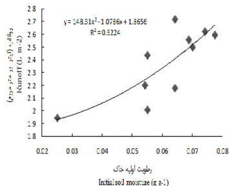
شکل ۷- رابطه بین رواناب و رطوبت اولیه در رخدادهای بارندگی
