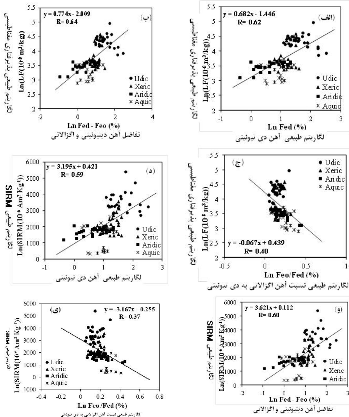
شکل ۲- پراکنش و معادلات رگرسیون خطی پذیرفتاری مغناطیسی در فرانس پایین (الف، ب، ج) و پسماند مغناطیسی اشباع (د، ه، و) در مقابل اشکال مختلف آهن
