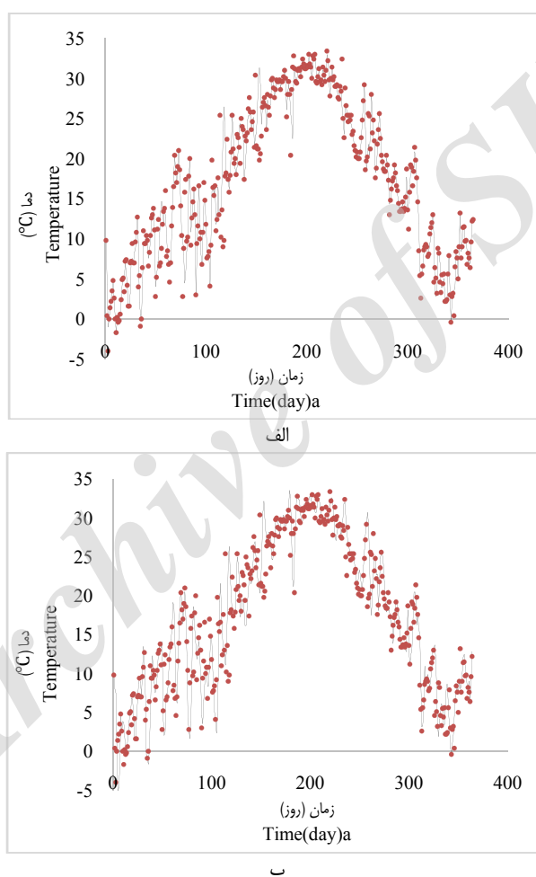
شکل ۴- دمای روزانه شبیه‌سازی شده‌ی سال ۲۰۰۹ با فاصله درون‌یابی ۱۰ روز و بدون استانداردسازی (الف) و با استانداردسازی (ب). دمای مدل‌سازی شده با خط ممتد و دمای اندازه‌گیری شده با نقطه نشان داده شده است
