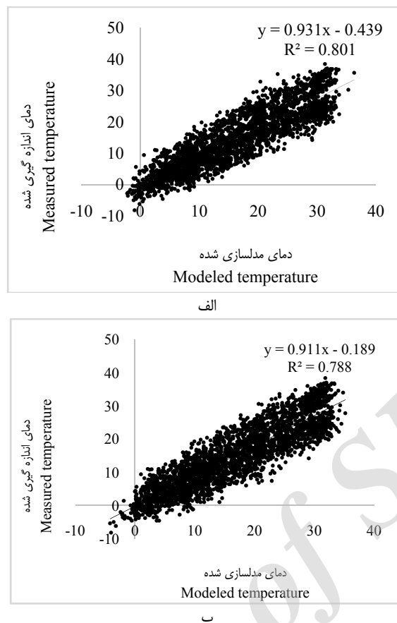
شکل ۸- مقایسه مقادیر دمای اندازه‌گیری شده با مقادیر شبیه‌سازی شده در مقیاس زمانی سه ساعته در سال ۲۰۰۹ با فاصله درون‌یابی ۵ روز الف: بدون استانداردسازی و ب: با استانداردسازی
