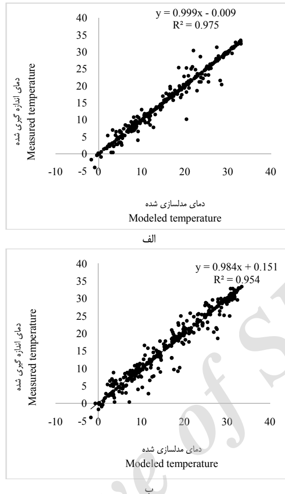
شکل ۵- مقایسه مقادیر دمای اندازه‌گیری شده با مقادیر شبیه‌سازی شده در مقیاس زمانی روزانه در سال ۲۰۰۹ با فاصله درونیابی ۵ روز و بدون استانداردسازی (الف) و با استانداردسازی (ب)
