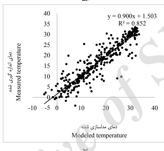
شکل ۶- مقایسه مقادیر دمای اندازه‌گیری شده با مقادیر شبیه‌سازی شده به روش فراکتال در مقیاس زمانی روزانه در سال ۲۰۰۹ با فاصله درون‌یابی ۱۰ روز و بدون استانداردسازی (الف) و با استانداردسازی (ب)
