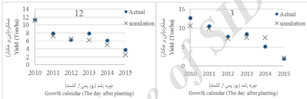
شکل 5- عملکرد واقعی و شبیه‌سازی شده سالانه طی سال‌های 2010 تا 2015 قطعات 3 و 12
