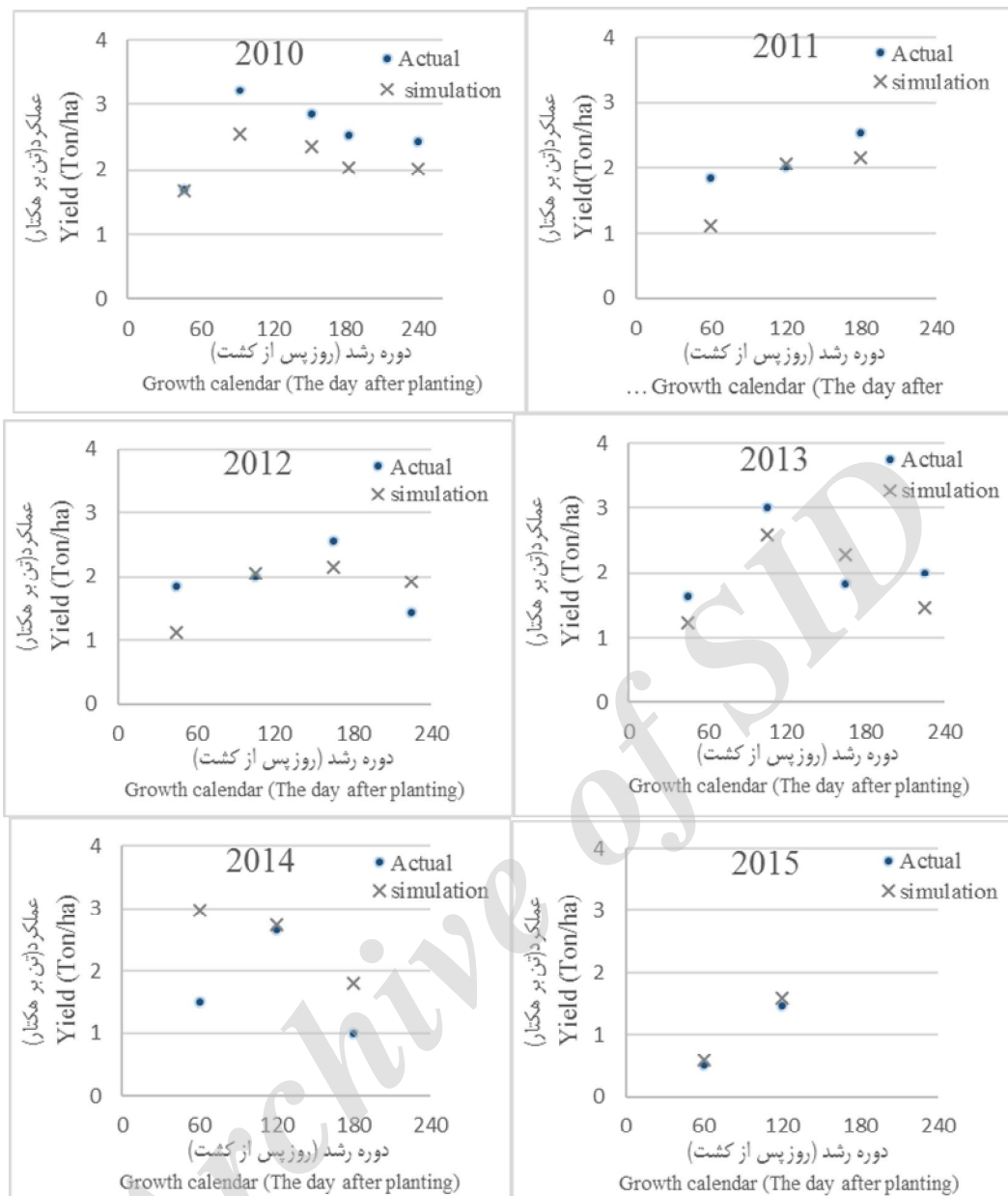
شکل 3- عملکرد واقعی و شبیه‌سازی شده طی سال‌های 2010 تا 2015 در برداشت‌های مختلف قطعه 3 Figure 3- Actual and simulated yields 2010 to 2015 in part 3
