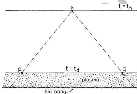
شکل ۴. دو نقطه p و q که در زمان جدایی ماده و تابش، بدون ارتباط علی بوده‌اند.
