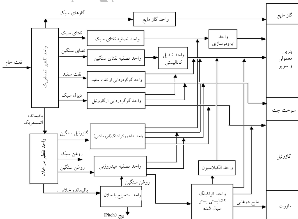
شکل ۱- شمای الگوی ۱ (کاهش باقی مانده های سنگین بر اساس فرایند استخراج با حلال و کراکنگ کاتالیستی)
