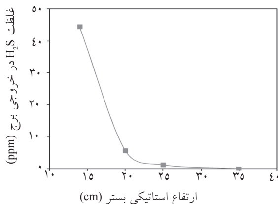
شکل ۸- تأثیر ارتفاع استاتیکی بستر بر میزان جذب گاز H 2 S (دبی گاز ۱۴۰۰ lit/hr، قطر آکنه ۲/۵ cm، دبی کاتالیست ۲۷ lit/hr و غلظت H 2 S در خوراک ۴۰۰۰ ppm)
