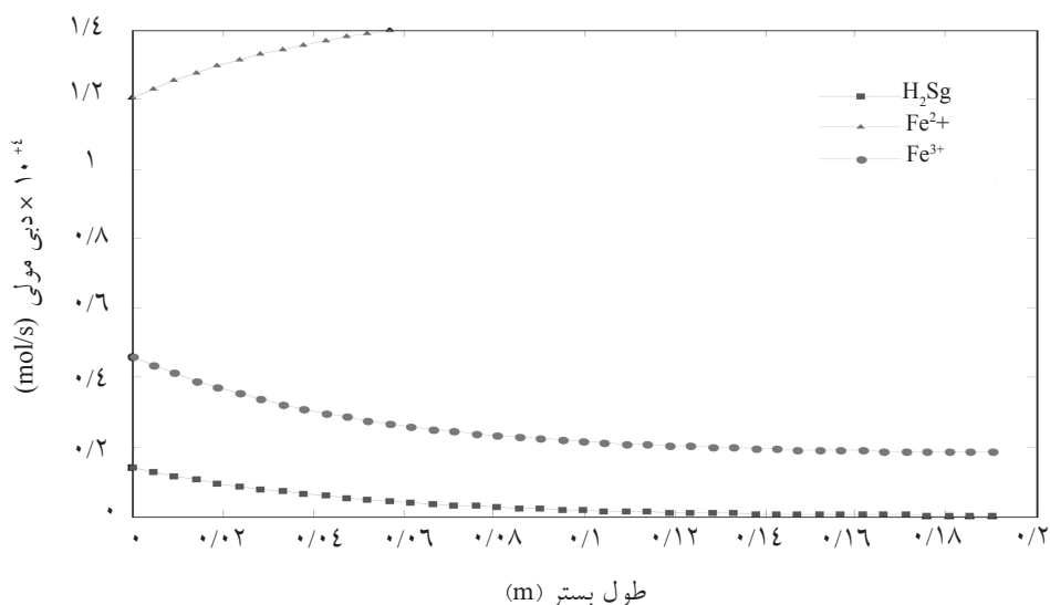
شکل ۴- تغییرات دبی مولی اجزاء مختلف در طول بستر برای آزمایش شماره ۸ جدول ۳- الف
