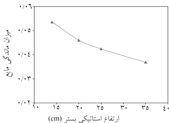
شکل ۱۰- تأثیر ارتفاع استاتیکی بستر بر میزان ماندگی مایع در برج (دبی گاز ۱۴۰۰ lit/hr، قطر آکنه ۲/۵ cm، دبی کاتالیست ۲۷ lit/hr و غلظت H 2 S در خوراک ۴۰۰۰ ppm)
