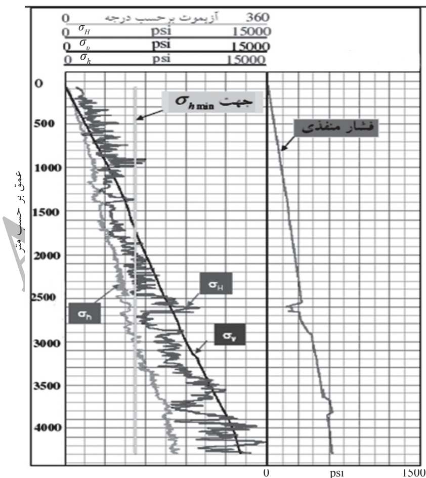
شکل ۲- پروفایل تنش‌های ( \sigma_H ، \sigma_v ، \sigma_h )، فشار منفذی و جهت \sigma_h در میدان مورد مطالعه [۵].
