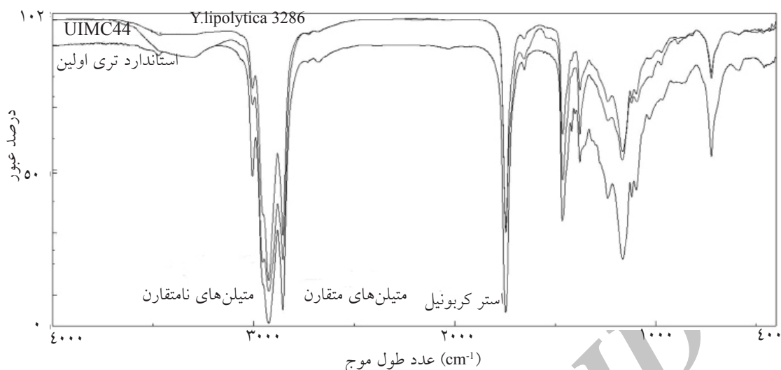
شکل ۷- گراف مربوط به تکنیک طیف‌سنجی مادون قرمز تبدیل فوریه، (سه گراف نشان‌داده شده در شکل مربوط به استاندارد تری اولین و روغن استخراج شده از دو سویه Y.lipolytica 3286 و UIMC44 می‌باشد).
