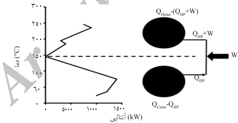
شکل ۶- انتگراسیون یک پمپ حرارتی در بالا و پایین پینچ
