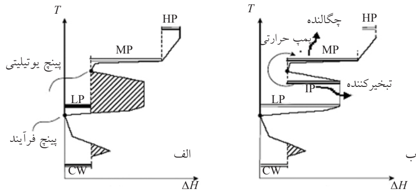
شکل ۷- قرارگیری مناسب یک پمپ حرارتی در بالا و پایین پینچ الف- منحنی مرکب کلی بدون پمپ حرارتی و ب- منحنی مرکب کلی با پمپ حرارتی [۱]
