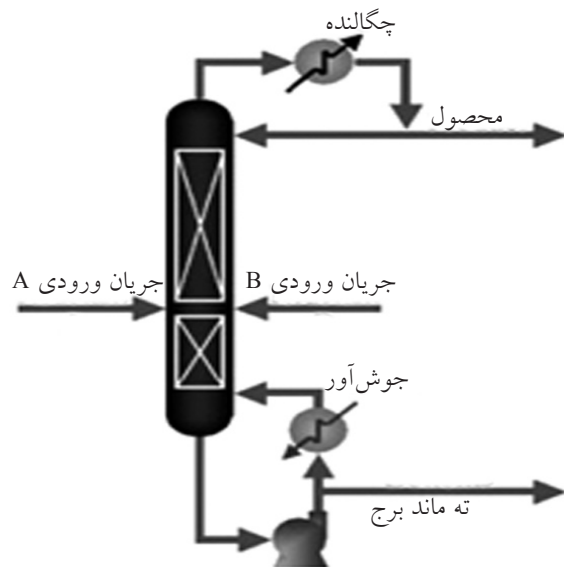
شکل ۲- یک واحد جداسازی معمولی بدون بازیافت انرژی
