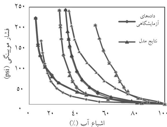
شکل ۶- مقایسه نتایج آزمایشات با نتایج مدل در نمونه‌های آسماری
