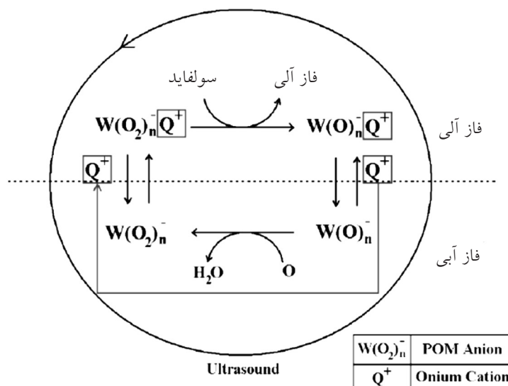
شکل ۲- شماتیک مدل اکسیداسیون کاتالیستی در فرآیند UAOD [۹] آنیون هتروپلی تنگستن با ساختار Keggin را نشان می‌دهد و Q^+ کاتیون چهارتایی آمونیومی می‌باشد
