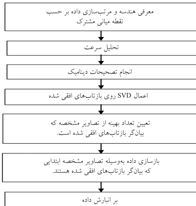
شکل ۵- طرح‌واره مربوط به مراحل تضعیف نوفه تصادفی با استفاده از تجزیه مقدار منفرد در داده نقطه عمقی مشترک.
