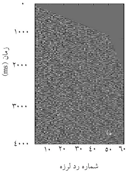
شکل ۹- الف) داده مصنوعی نقطه عمقی مشترک تولید شده با نسبت سیگنال به نوفه ۱، ب) داده پس از تحلیل سرعت مناسب و اعمال تصحیحات دینامیک، ج) نمودار مقادیر ویژه در مقابل اندیس آن برای شکل ب، د) داده فیلتر شده و ه) اختلاف بین داده فیلتر شده و ورودی
