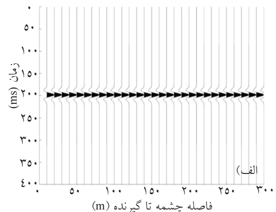
شکل ۱-الف) یک پدیده لرزه ای افقی با فرکانس مرکزی ۱۰ Hz در ۳۰ ردلرزه با فاصله ۱۰ m، نسبت سیگنال به نوفه بی نهایت و زمان نمونه گیری ۲ ms (ب) مقادیر ویژه در مقابل اندیس آن برای پدیده (الف).
