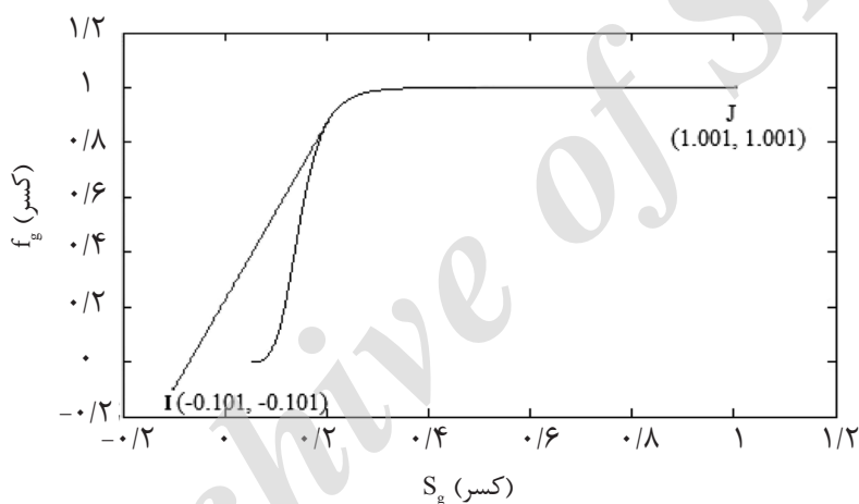
شکل ۷ تعیین اشباع نواحی مدل In-house با روش ترسیم I-J.
