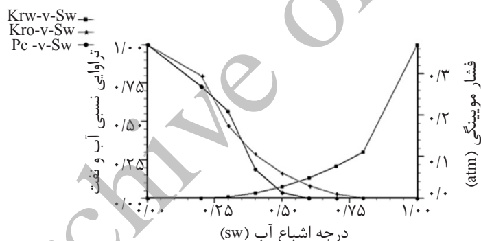
شکل ۲- توابع استفاده شده برای تراوایی نسبی و فشار موئینگی [۱۶]
