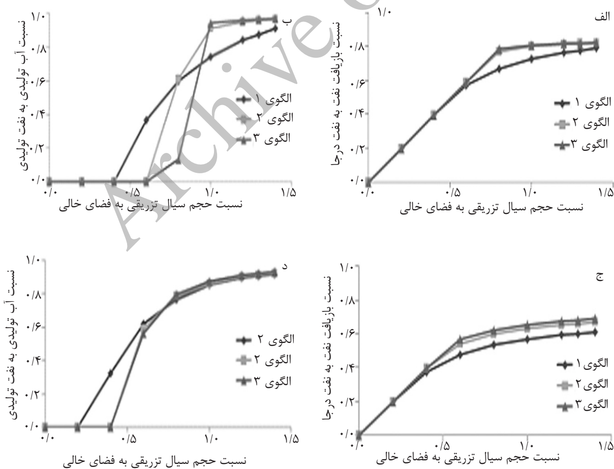
شکل ۱۰- نمودارهای بررسی اثر زاویه شکاف در الگوهای الف، د و ه. (الف) باز یافت نفت در تزریق پلیمر، (ب) برش آب در تزریق پلیمر، (ج) باز یافت نفت در تزریق آب، (د) برش آب در تزریق آب
