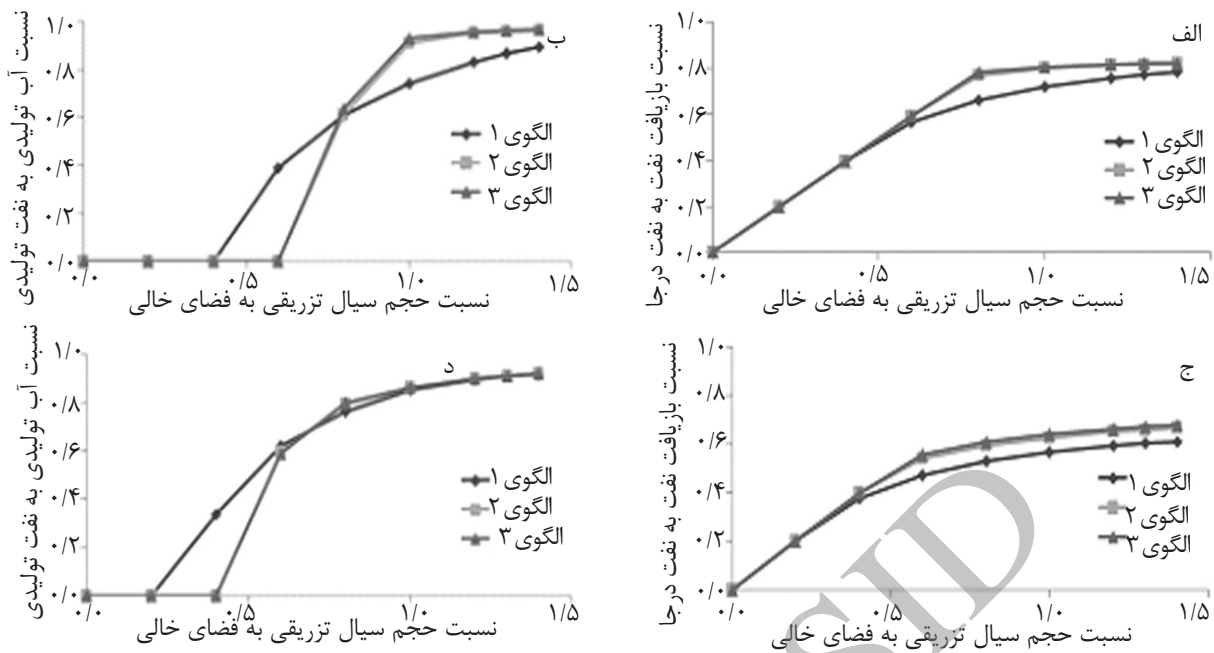
شکل ۸- نمودارهای بررسی تأثیر طول شکاف در الگوهای الف، ب و ج. (الف) بازیافت نفت در تزریق پلیمر، (ب) برش آب در تزریق پلیمر، (ج) بازیافت نفت در تزریق آب، (د) برش آب در تزریق آب (الگوهای ۲ و ۳ هم‌پوشانی دارند)
