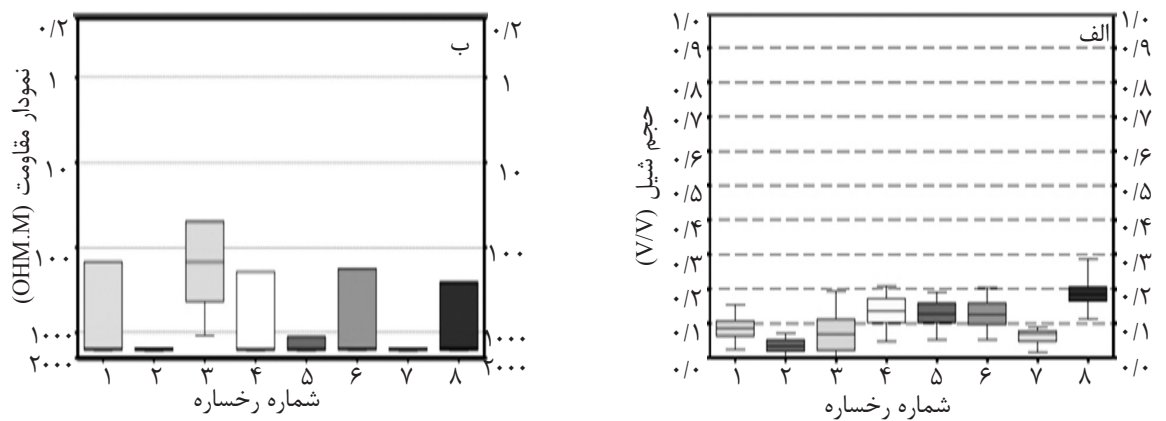
شکل ۵- نمودارهای حجم شیل (الف) و نمودار مقاومت (ب) در رخساره‌های شناسایی شده توسط روش آنالیز خوشه‌ای در چاه B
