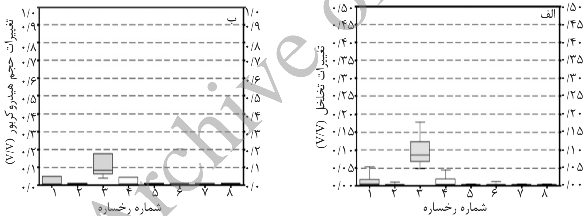
شکل ۴- نمودارهای تخلخل (الف) و حجم هیدروکربور (ب) در رخساره‌های شناسایی شده توسط روش آنالیز خوشه‌ای در چاه B
