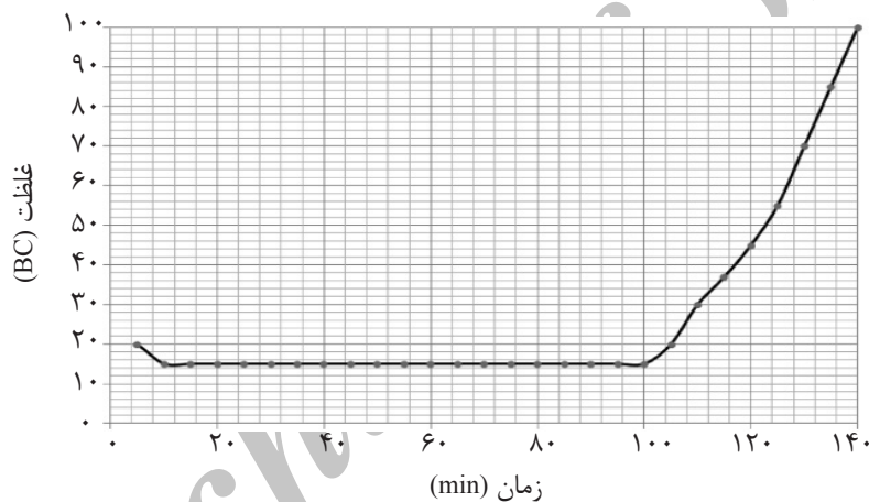
شکل ۳- آزمایش زمان نیم بندش دوغاب سیمان شماره ۶
