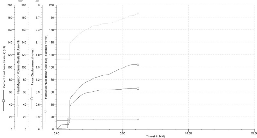
شکل ۷- تغییرات حجم سیال نفوذی به داخل دوغاب سیمان و صافاب خارج شده از آن در تست مهاجرت گاز
