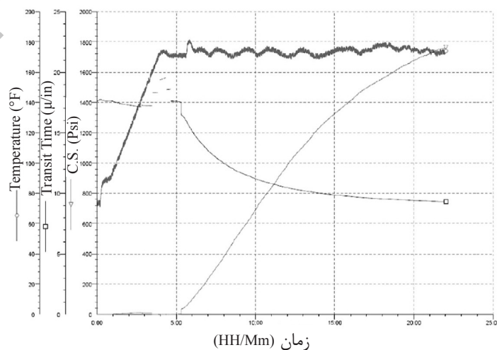
شکل ۴- الگوی توسعه مقاومت فشاری دوغاب سیمان شماره ۶
