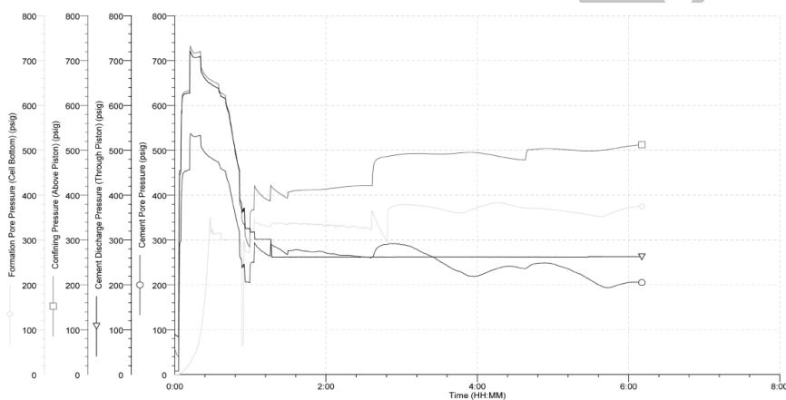
شکل ۶- تغییرات فشار منفذی و فشار تزریق گاز دوغاب سیمان طی آزمایش مهاجرت گاز
