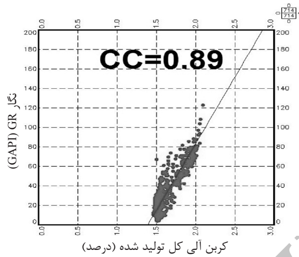
شکل ۱۱- نمودار متقاطع TOC تولید شده در برابر نگار GR
