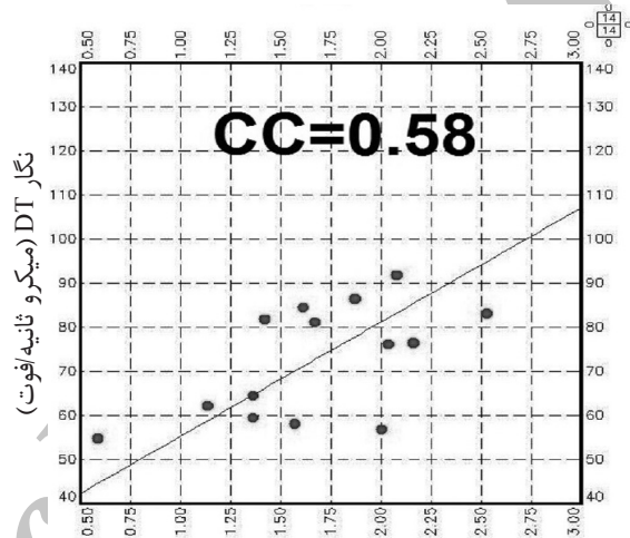
شکل ۵- نمودار متقاطع DT در برابر کربن آلی کل
