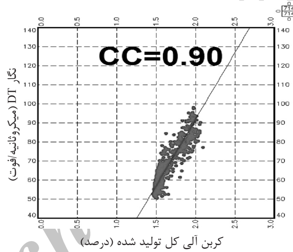
شکل ۱۲- نمودار متقاطع TOC تولید شده در برابر نگار DT
