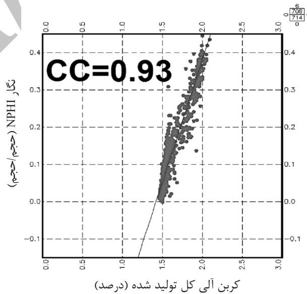
شکل ۱۳- نمودار متقاطع TOC تولید شده در برابر نگار NPHI
