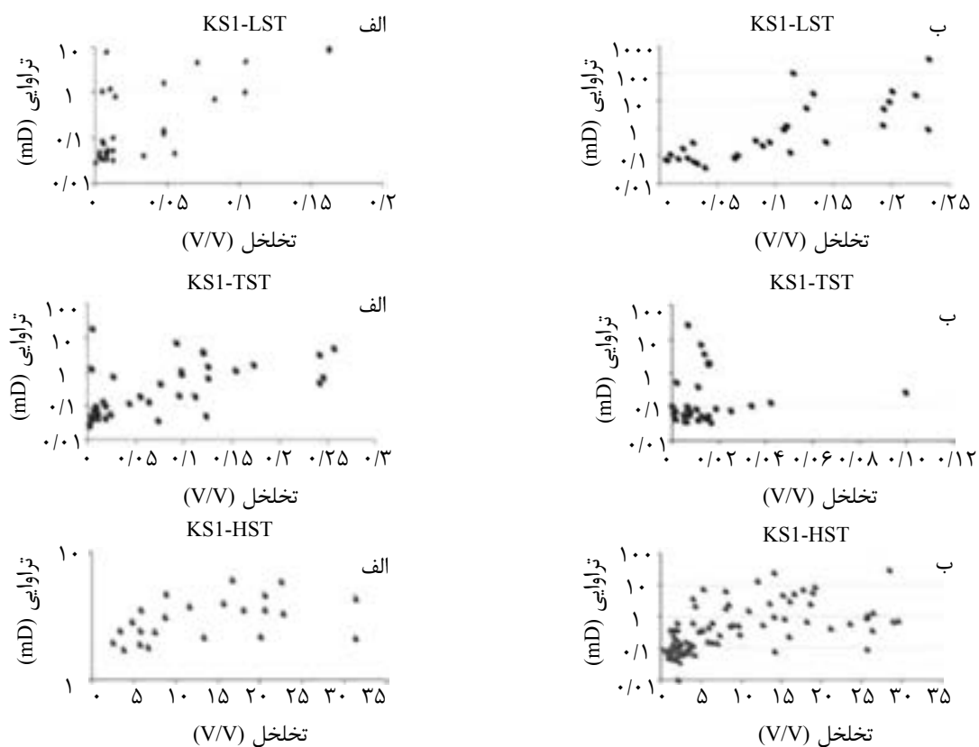
شکل ۵ نمودار توزیع داده‌های تخلخل و تراوایی در چاه SP-A (الف) و SP-B (ب) در سکناس KS1.
