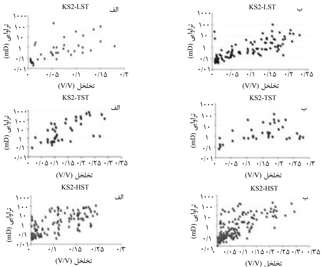
شکل ۴ نمودار توزیع داده‌های تخلخل و تراوایی در چاه SP-A (الف) و SP-B (ب) در سکناس KS2.
