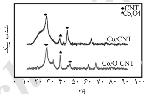
شکل ۳- پراش اشعه ایکس Co/CNT و Co/O-CNT
