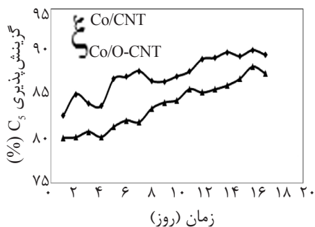
شکل ۹- تغییرات گزینش پذیری محصولات مایع با زمان
