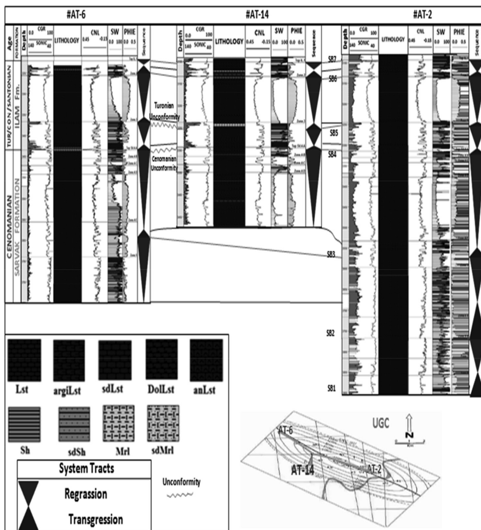
شکل ۳ تطابق چینهننگاری سکansı بین چاههای شماره ۲، ۶ و ۱۴ میدان آبتیمور
