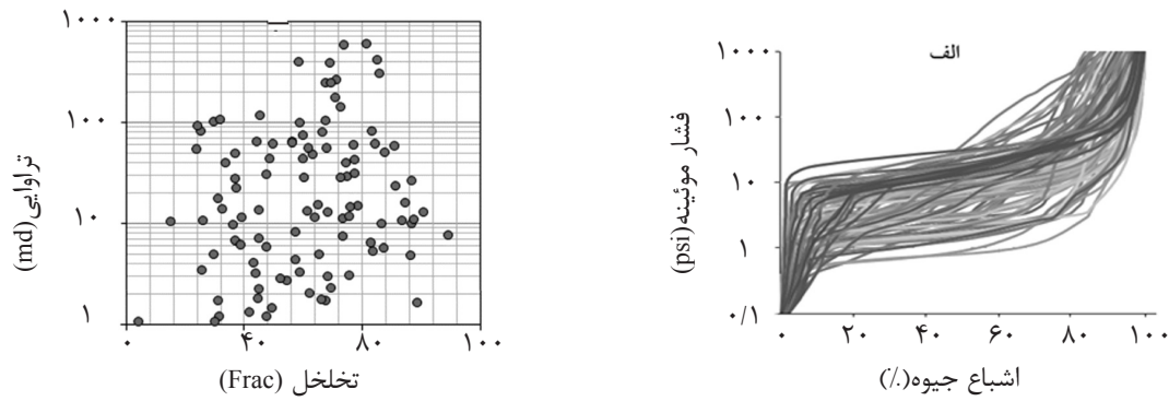
شکل ۳ الف) نمودار فشار تزریق جیوه در مقابل اشباع‌شدگی نمونه‌ها و ب) نمودار تخلخل در مقابل تراوایی نمونه‌ها.
