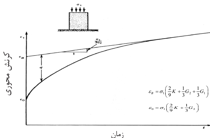
شکل ۷ خزش در فشار تک محوره سنگی که تحت مدل برگر رفتار می کند [۱۲].
