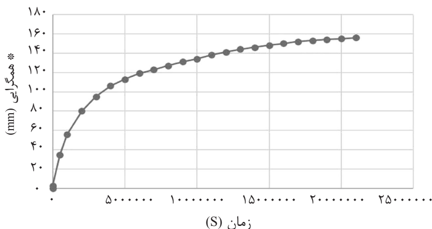
شکل ۹- همگرایی دیواره چاه بدون حضور سیال حفاری. * اختلاف قطر اولیه چاه و قطر چاه بعد از تغییر شکل تقسیم بر ۲
