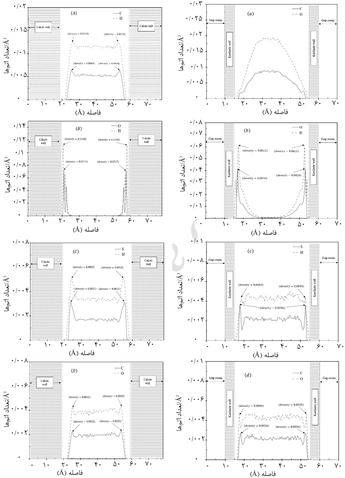
شکل ۴ توزیع دانسیته جذب در سیستم‌های (A) M-Calcite-C 10 , (B) M-Calcite-H 2 O , (C) M-Calcite-H 2 S , (D) M-Calcite-CO 2 , (a) M-Kaolinite-C 10 , (b) M-Kaolinite-H 2 O , (c) M-Kaolinite-H 2 S , (d) M-Kaolinite-CO 2 در هر محور عمودی معرف دانسیته در هر آنگستروم مکعب و محور افقی معرف فاصله بر حسب آنگستروم می‌باشد.
