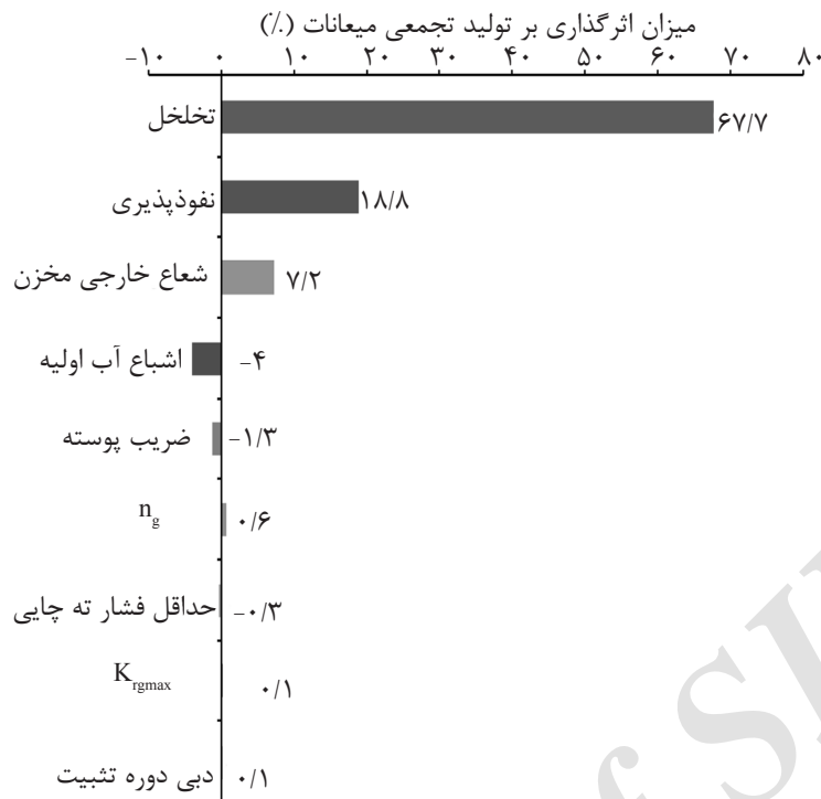
شکل ۴ نمودار تورنادو برای نشان دادن اثر عدم قطعیت در هر یک از داده‌های ورودی بر تولید میعانات تجمعی برای چاه عمودی.
