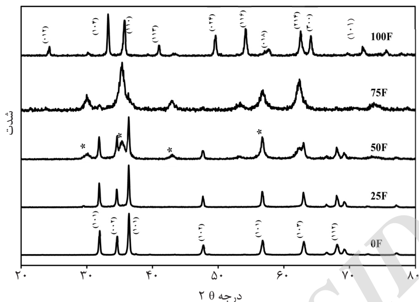
شکل ۲ نمودار XRD نمونه‌ها که علامت * بر روی قله‌های نمونه 50F بیانگر قله‌های مربوط به ZnFe_2O_4 است.
