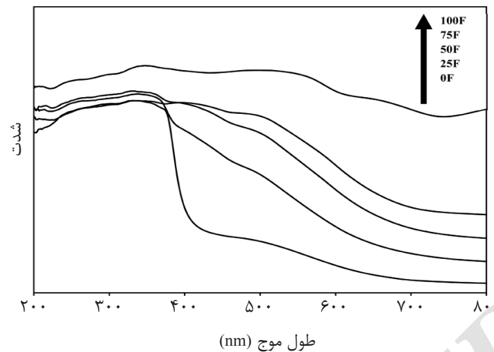
شکل ۵ نمودار طیف UV-vis نمونه‌ها.
