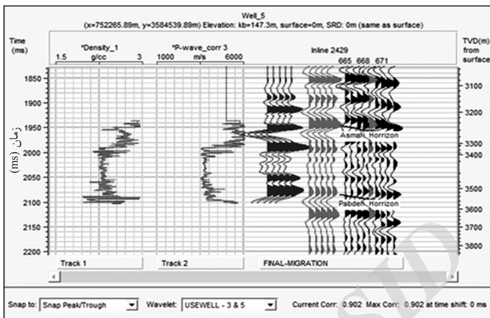
شکل ۵ پنجره‌ای از ارتباط دادن داده لرزه‌ای (گره زدن) به وسیله لرزه نگاشت مصنوعی در چاه شماره ۵.
