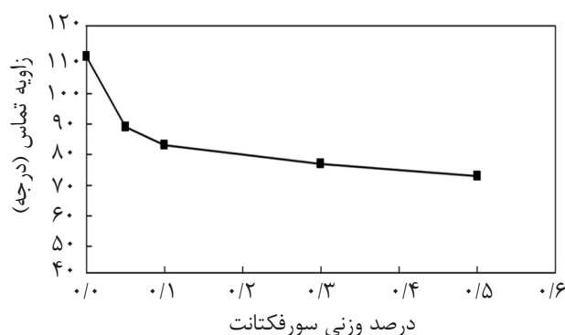
شکل ۳ تأثیر غلظت سورفکتانت دودسیل تری متیل آمونیوم برمید بدون حضور ماده قلیایی بر کاهش زاویه تماس
