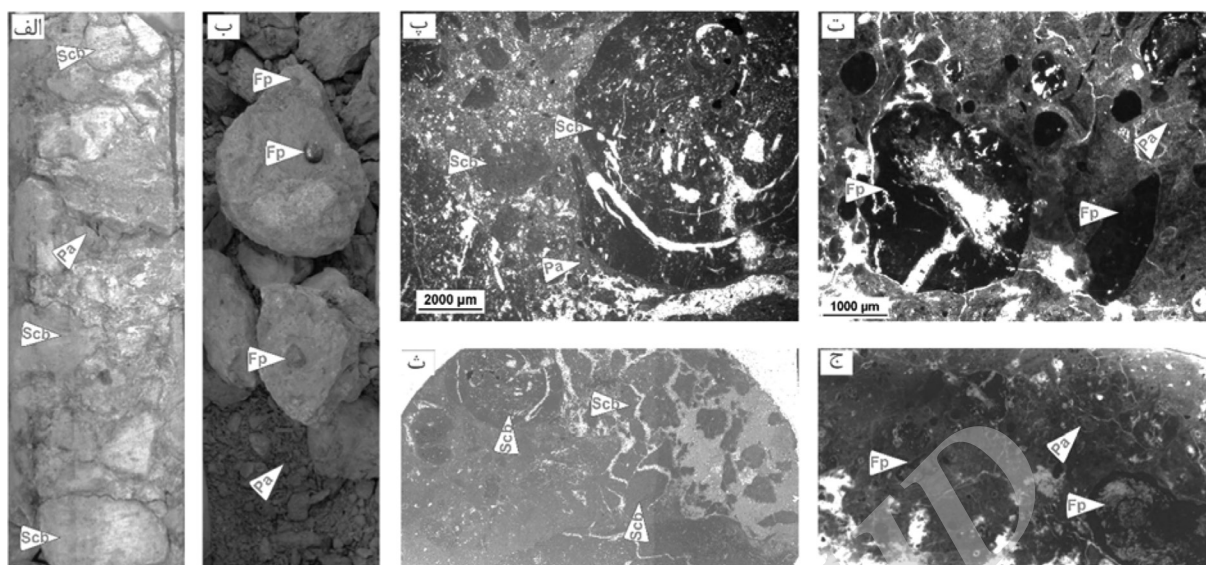
شکل ۲ تصاویر مغزه (الف-ب)، مقاطع نازک میکروسکوپی (پ-ت) و اسکن آنها (ث-ج) از شواهد دو سطح ناپیوستگی در بخش بالایی سازند سروک. الف-پ-ث) ناپیوستگی مرز سنومانین-تورونین، (ب-ت-ج) ناپیوستگی تورونین میانی، علائم اختصاری (Fp): پیژولیت آهن، Scb: خاک قدیمه، Pa: خاک قدیمه
