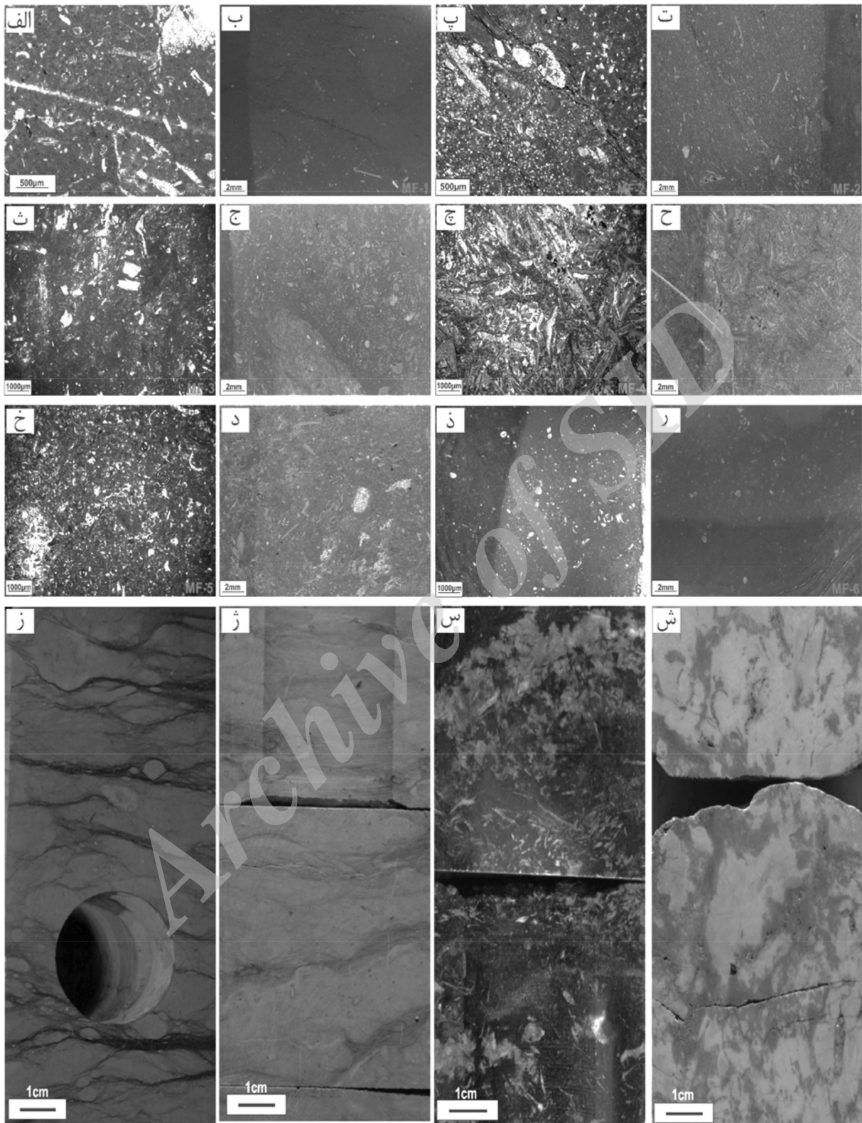
شکل ۳ تصاویر مقاطع نازک میکروسکوپی، (الف-پ-ث-چ-خ-ذ) اسکن مقاطع (ب-ت-ج-ح-د-ر) به همراه تصاویر مغزه (ز-ژ-س-ش) از رخساره‌های شناسایی شده در سازند سروک براساس داده‌های در دسترس: الف-ج-ز) مادستون- وکستون الیگوستژین دار (MF-1)، پ-ت)، وکستون اکینودرم دار (MF-2)، ث-ج-ژ) وکستون-فلوتستون دارای خرده‌های رودیستی (MF-3)، چ-ح) پکستون-رودستون با واریزه رودیستی (MF-4)، خ-د-س) وکستون-پکستون دارای فرامینفرهای بنتیک (MF-5)، ذ-ر-ش) مادستون- وکستون میلیولید دار (MF-6). تصاویر مقاطع نازک پ-چ-ذ در XPL و سایر تصاویر در PPL
