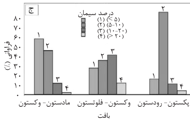
شکل ۷ الف) نمودار فرآوانی سیمان کلسیتی درون رخساره‌های مخزن با توجه به نوع حفرات، ب) منافذ پر شده با سیمان براساس درصد‌های حجمی مختلف، پ) فرآوانی هر کدام از گروه‌های درصد حجمی در ارتباط با بافت سنگ
