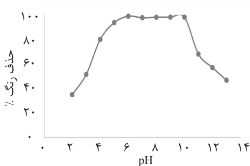
شکل ۵ اثر pH محلول بر میزان بازیابی متیلن بلو از 20/0 cc محلول حاوی 8/5 mg متیلن بلو
