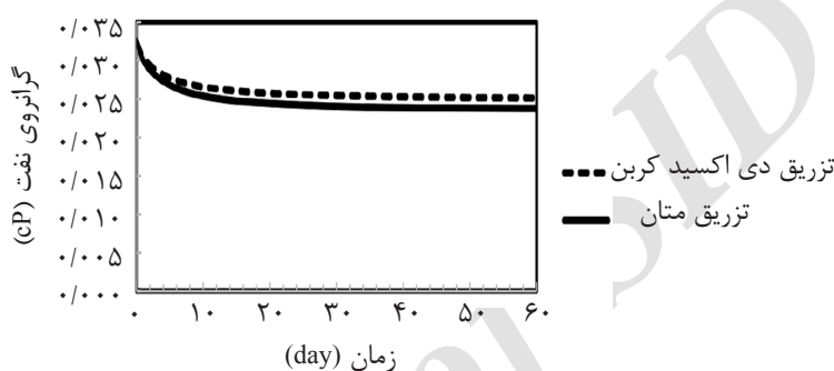
شکل ۱۱ تغییرات گرانروی نفت موجود در ماتریس حین تزریق گاز دی اکسید کربن و متان با مدل فیک تعمیم یافته
