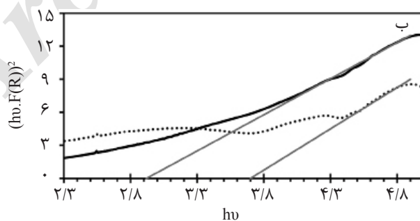
شکل ۵ نمودار آنالیز UV-vis مربوط به نمونه \text{TiO}_2 قبل و بعد از داپ با نیتروژن و (ب) نمودار hv برحسب (hv * F(R))^2 برای محاسبه طول شکاف نوار
