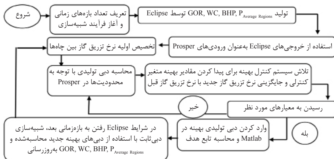
شکل ۴ فلوجارت تخصیص بهینه گاز تزرفی بین چاه‌ها
