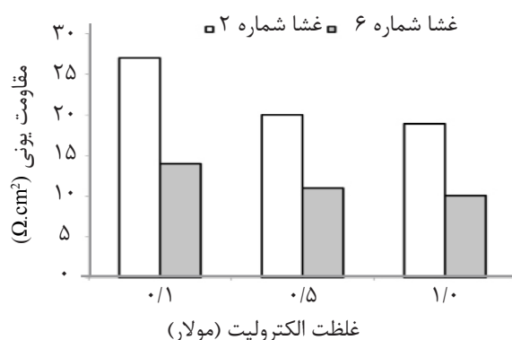
شکل ۶ بررسی اثر غلظت و pH محلول الکترولیت بر مقاومت یونی غشاها
