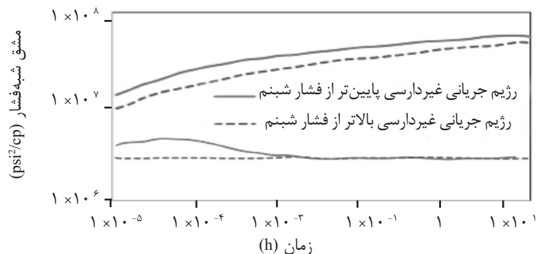
شکل ۱۰ نمودارهای ساخت فشار لگاریتمی - لگاریتمی شبه فشار و مشتق شبه فشار نسبت به زمان برای رژیم جریان غیرداری در فشار بالاتر و پایین تر از فشار نقطه شبنم
