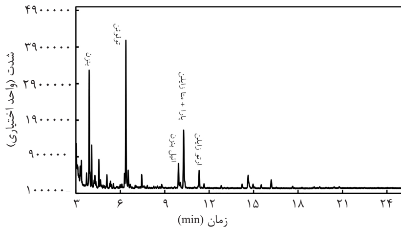
شکل ۲ کروماتوگرام به‌دست آمده از دستگاه GC-MS جهت شناسایی ترکیبات BTEXs در نمونه استخراجی از خودروی پژو ۴۰۵
