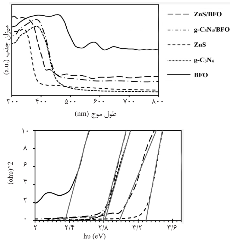
شکل ۴ الف) طیف جذب UV-Vis فتو کاتالیست‌های سنتز شده. ب) تخمین شکاف باند فتوکاتالیست‌های سنتز شده
