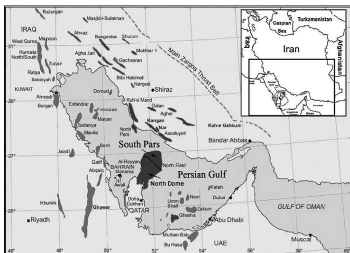
شکل ۱ نقشه جغرافیایی میداین هیدروکربوری خلیج فارس و توالی چینه‌شناسی منطقه مورد مطالعه
