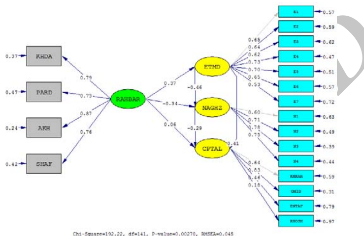
شکل ۱. مدل معادلات ساختاری در حالت تخمین استاندارد
