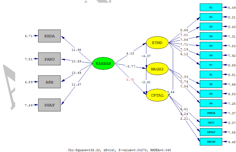
شکل ۲. مدل معادلات ساختاری در حالت اعداد معناداری
