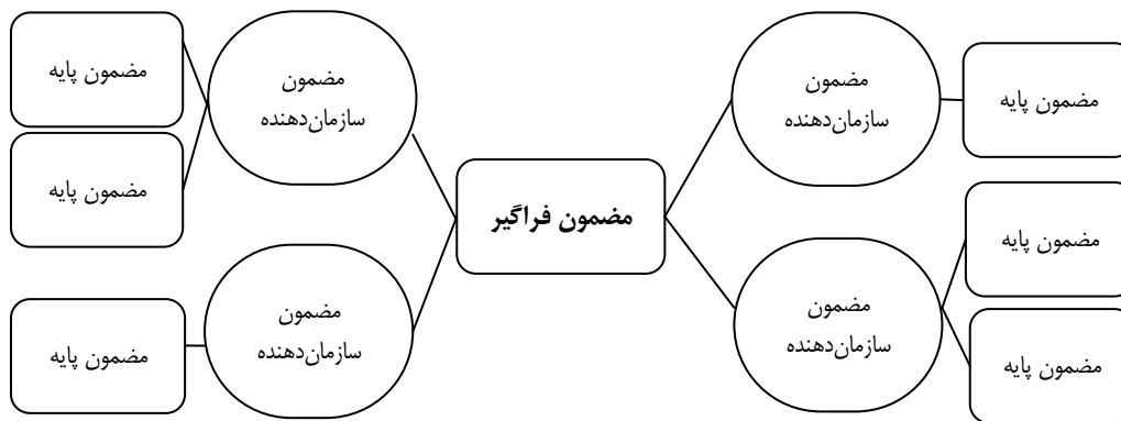
شکل ۱: شبکه مضمون‌ها
