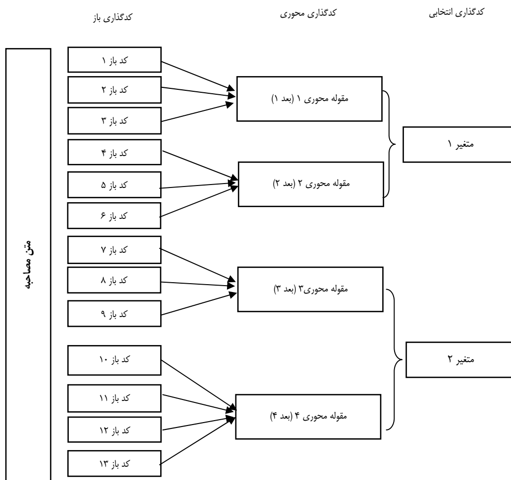
شکل ۱. مراحل کدگذاری
