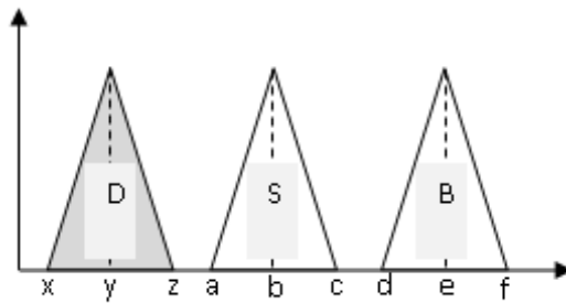
نمودار ۵. رابطه خواست تصمیم گیرنده و عملکرد گزینه در حالت تکنیک تخصیص بدیهی سنتی
