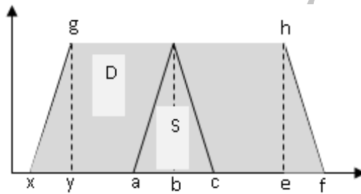
نمودار ۶. رابطه خواست تصمیم گیرنده و عملکرد گزینه در حالت تکنیک تخصیص بدیهی بهبود یافته
